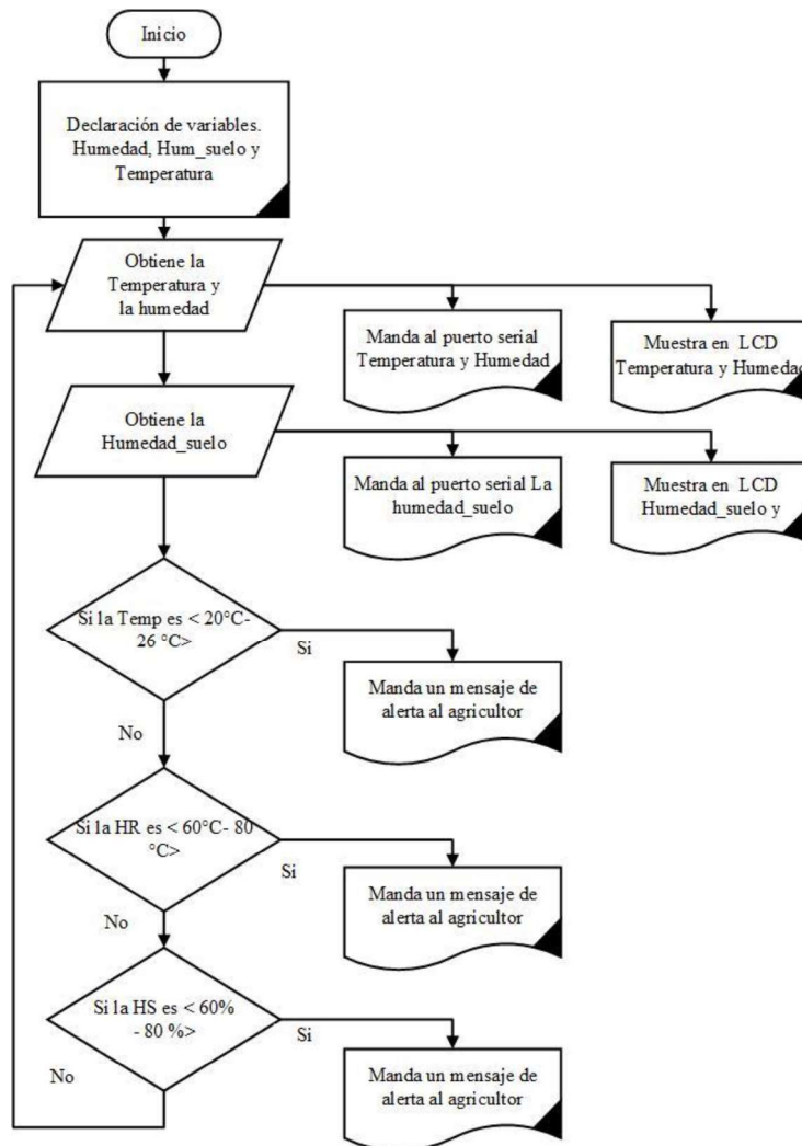
Figura 2. Diagrama de flujo para Arduino
