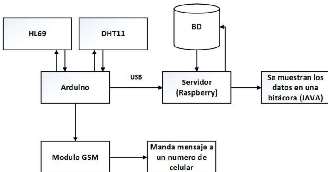
Figura 1. Diagrama a bloques
